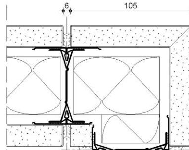
Ecke M 1:2
